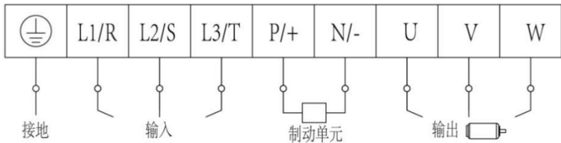
图 4-7 端子示意图
